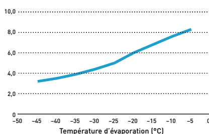
OCU-CR400VF8A(SL) 2) Puissance frigorifique (kW)
