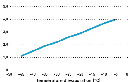
OCU-CR200VF5A(SL) 1) Puissance frigorifique (kW)
