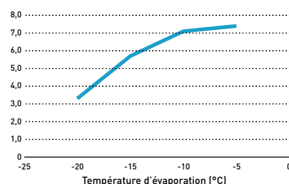
OCU-CR400VF8(SL) 2) Puissance frigorifique (kW)
