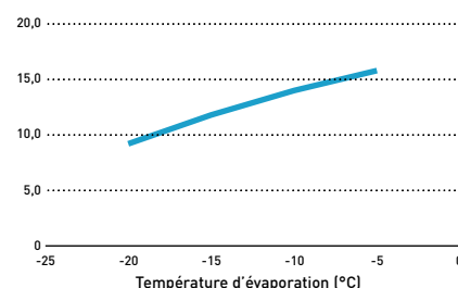
OCU-CR1000VF8(SL) 2) Puissance frigorifique (kW)
