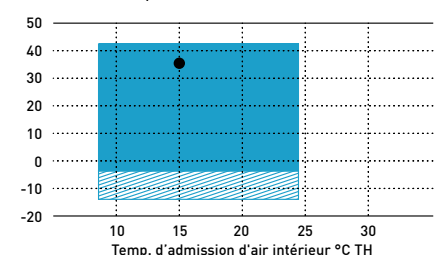
Plage de températures pour cave à vin. En mode froid. Temp. d'admission d'air extérieur °C TS.
